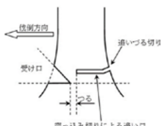
図4 追いづる切り
