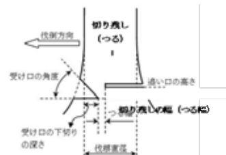
図 2 受け口、小井口及び切り残し（つる）の関係
